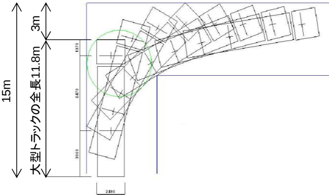
（大型トラックの旋回軌跡図）
